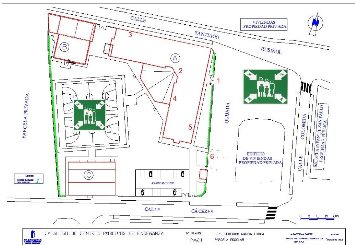
Plano de Evacuación General IES nº8.
